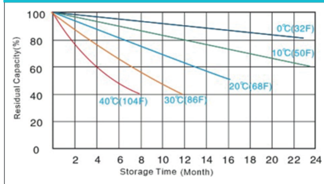
Характеристики хранения
