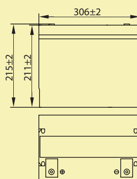
РАЗМЕРЫ
