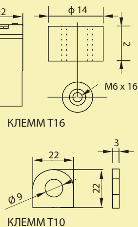
ТИП КЛЕММ
